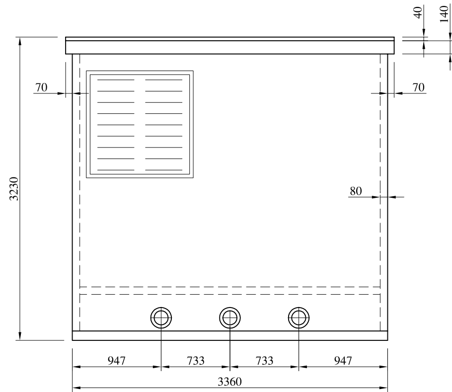
VISTA POSTERIOR
