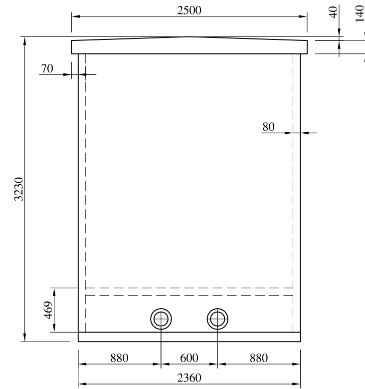
VISTA LATERAL
