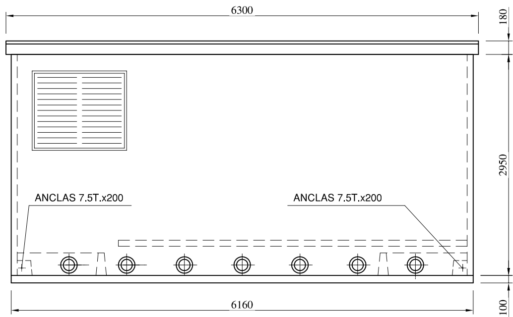
VISTA POSTERIOR
