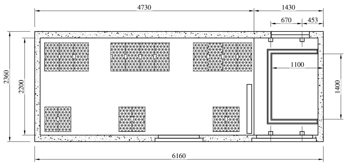
SECCION A
