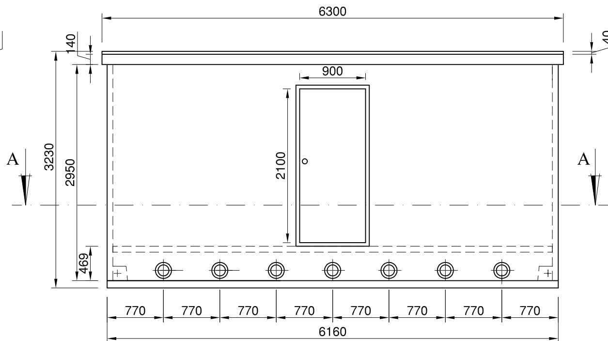
CARA FRONTAL
