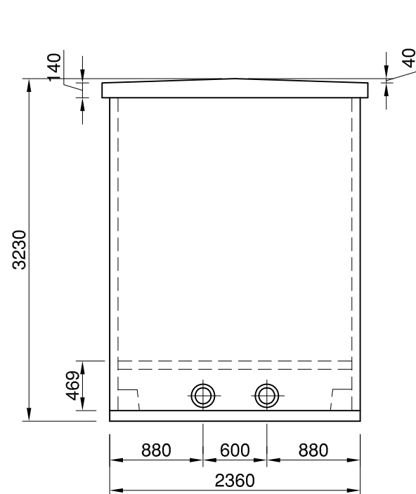
CARA IZQUIERDA
