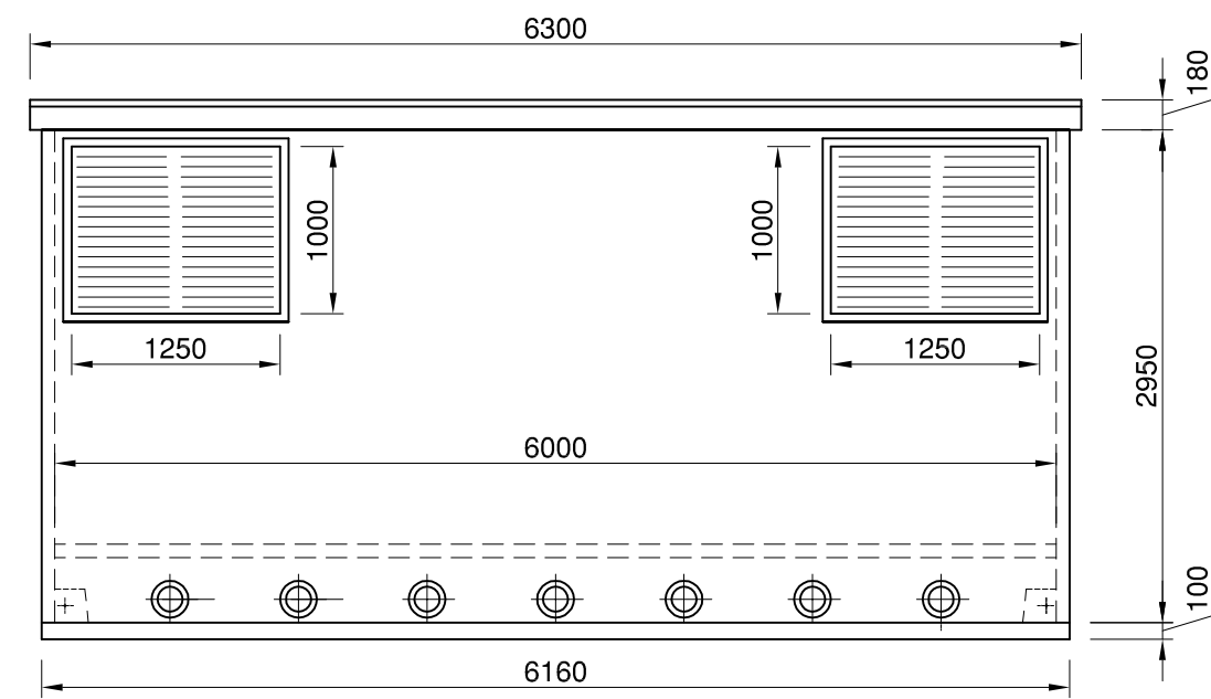
CARA POSTERIOR
