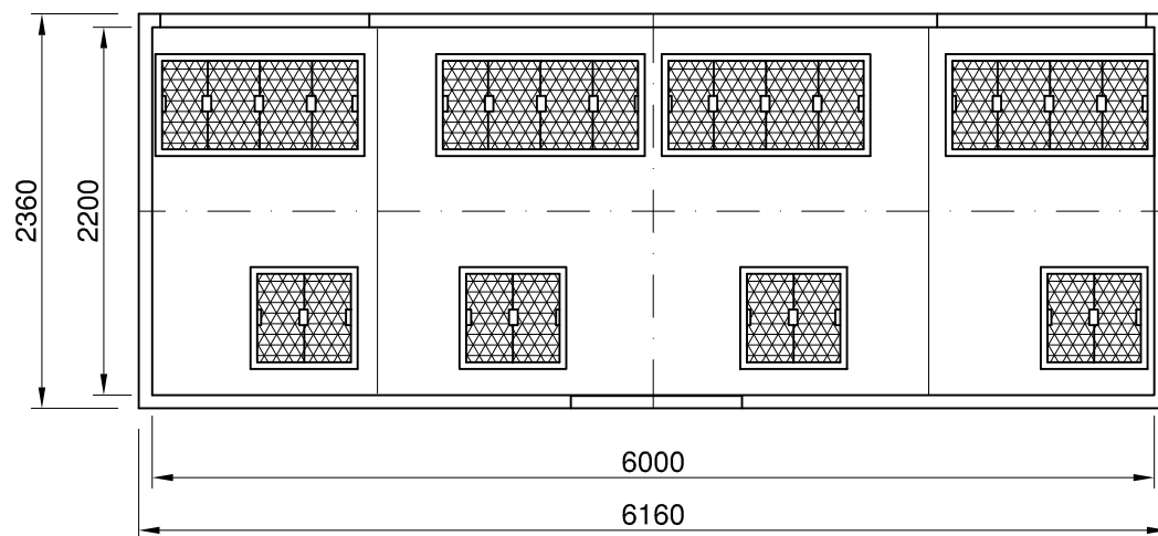
SECCION A-A
