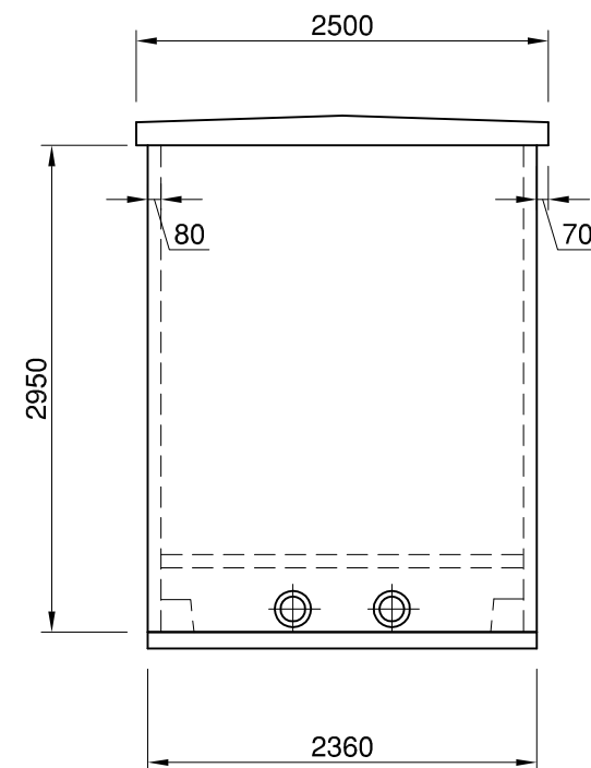
CARA DERECHA
