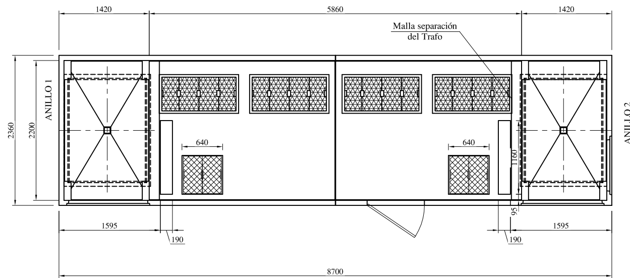
SECCION A-A (LOSA SUPERIOR)
