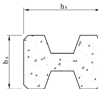
SECCION B-B
