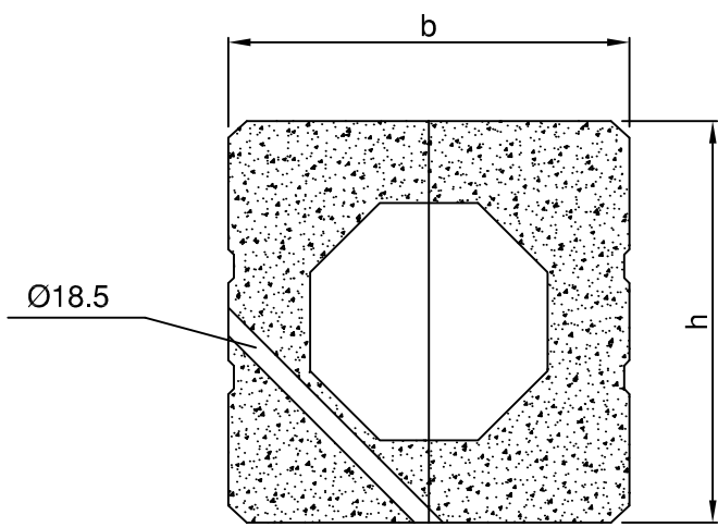
SECCION B-B
